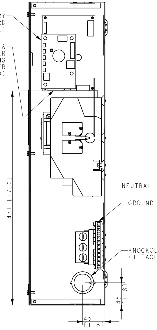
SECTION A-A
